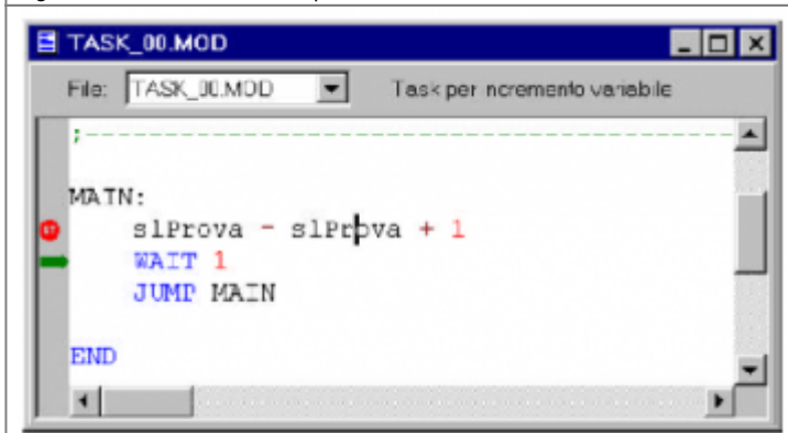
Figura 37: inserimento breakpoint.
