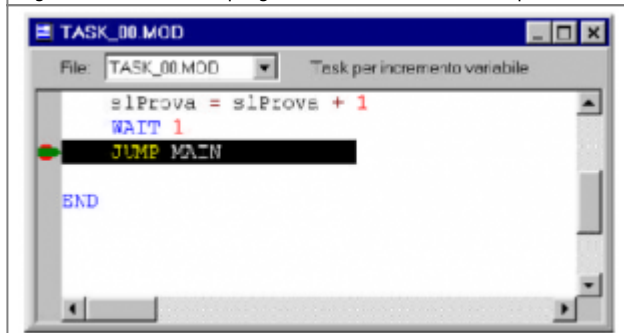
Figura 23: esecuzione programma interrotta da breakpoint.
