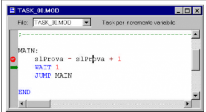
Figura 37: inserimento breakpoint.
