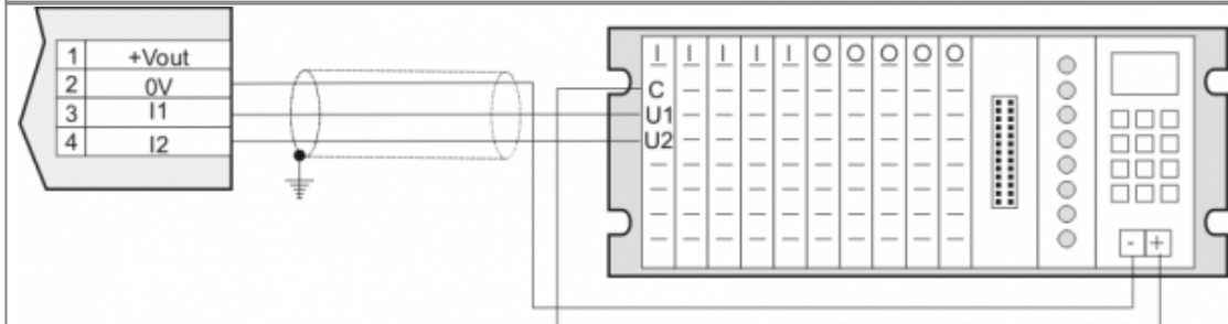
Ingressi digitali PNP collegati ed alimentati (Vdc) da PLC.
