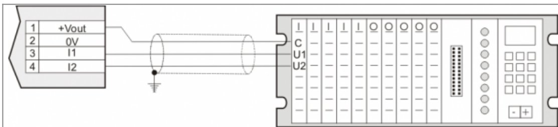
Ingressi digitali PNP collegati a PLC alimentati da MC135.
