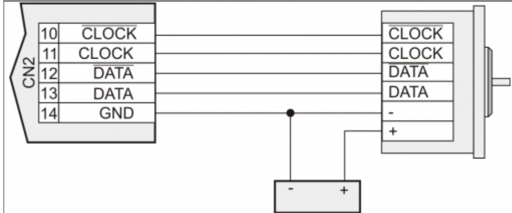
Collegamento Encoder SSI alimentato da un alimentatore esterno
