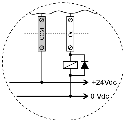
Esempio di collegamento con relè DC Connection example with DC relay
