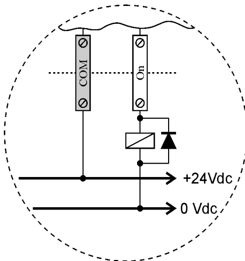
Esempio di collegamento con relè DC Connection example with DC relay
