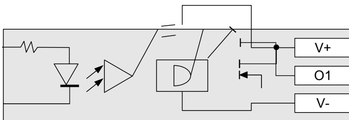
Fig. 2: Schema elettrico / Electric layout
